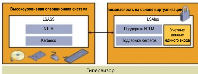
Рис. 4-1. Процесс LSA на основе виртуализации.
