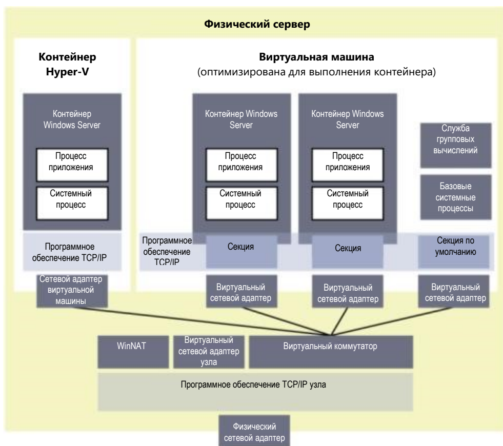
Рис. 3-11. Сетевые подключения контейнеров
