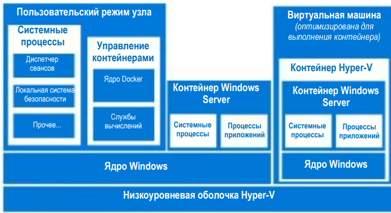
Рис. 3-7. Контейнеры Windows Server 2016 и контейнеры Hyper-V на одном и том же физическом сервере Как показано на рисунке, на одном физическом сервере может одновременно использоваться целый набор из контейнеров Hyper-V, виртуальных машин и контейнеров Windows Server. Поскольку доступны два типа контейнеров, возникает вопрос, в каких случаях для разработки и развертывания приложений следует использовать контейнеры Windows Server, а в каких — контейнеры Hyper-V. Выбор зависит от требований приложения (или заказчика, использующего контейнеры) к масштабированию и изоляции с аппаратной поддержкой.
