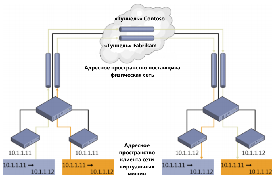
Рисунок 2-67. Адресные пространства.
