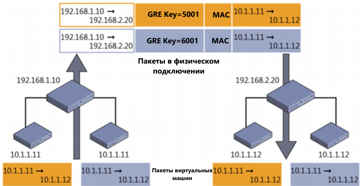
Рисунок 2-68. Инкапсуляция маршрутов при виртуализации сети (NVGRE).
