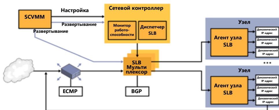
Рисунок 2-70. Общее устройство программного балансировщика нагрузки.
